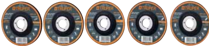
ABT-386 ABT-774 ABT-556 ABT-390 ABT-754
