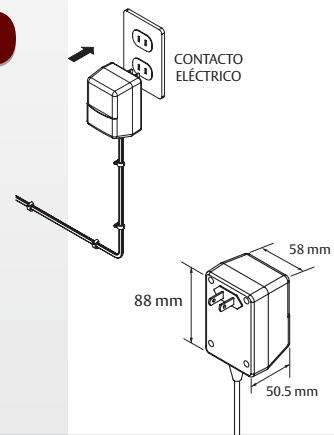
Mod. HA48N8250 IDEAL PARA CERRADURA 321 Y CONTRA 310
